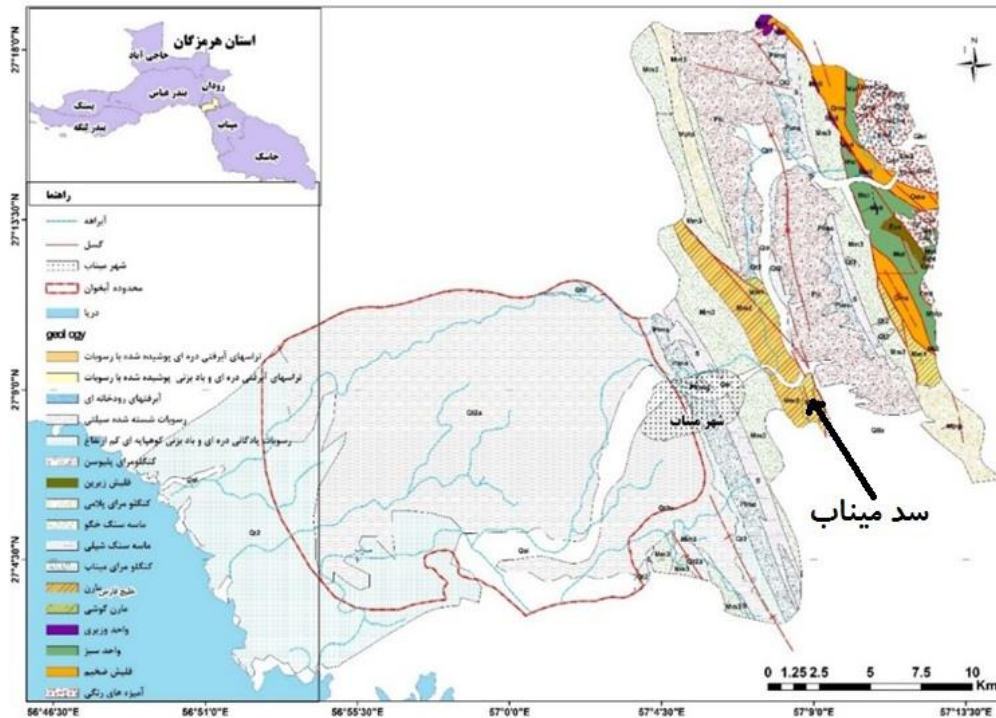
شکل ۱- موقعیت و وضعیت زمین‌شناسی محدوده مطالعاتی میناب (تهیه شده بر اساس نقشه ۱:۱۰۰,۰۰۰ میناب)
