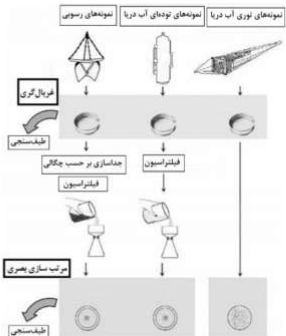
شکل ۳- روش‌های مختلف نمونه‌برداری از میکروپلاستیکها در محیط‌های مختلف و مراحل پردازش نمونه‌ها (Ruz et al. 2012) Fig. 3 Different methods of sampling microplasmas in different environments and process stages of samples (Ruz et al. 2012)
