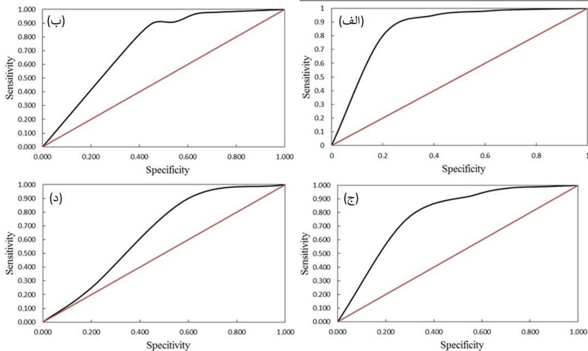
شکل ۴ منحنی‌های ROC برای استان‌های الف- استان آذربایجان شرقی، ب- استان آذربایجان غربی، ج- کردستان، و د- اردبیل Fig. 4 ROC Curves for: a) East Azerbaijan, b) West Azerbaijan, c) Kurdistan, and d) Ardabil provinces
