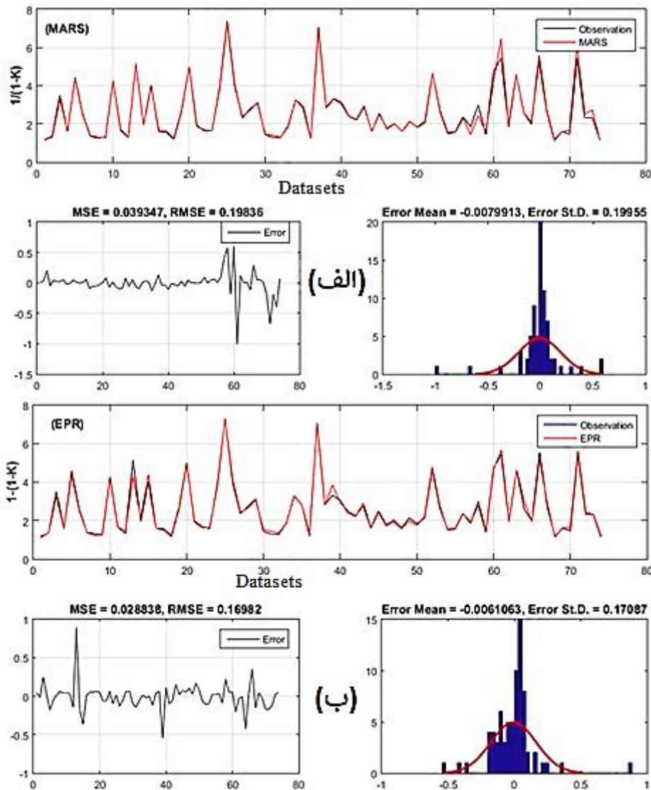
شکل ۴- مقادیر افت انرژی مشاهداتی و پیش‌بینی‌شده توسط مدل‌های محاسبات نرم مورد استفاده برای کل داده‌های مراحل آموزش و آزمایش: الف- مدل MARS، و ب- مدل EPR
