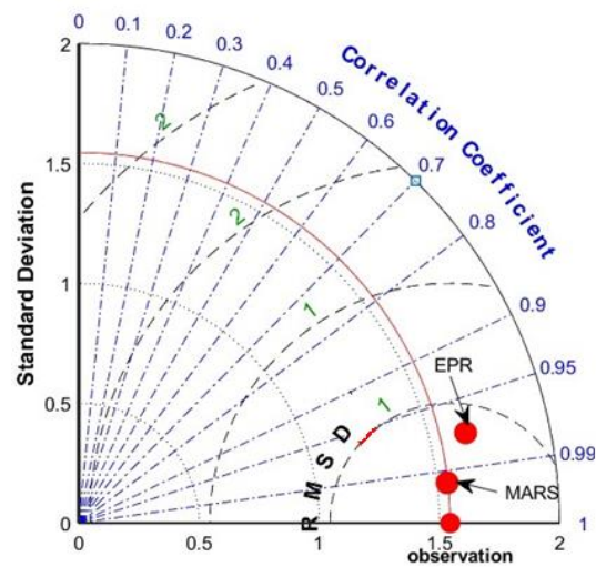
شکل ۲- دیاگرام تیلور
