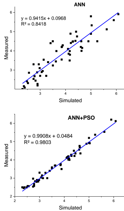
شکل ۶- نمودار پراکندگی داده‌های اندازه‌گیری و شبیه‌سازی برای پارامتر کیفی SAR بر حسب \text{mg/l}
