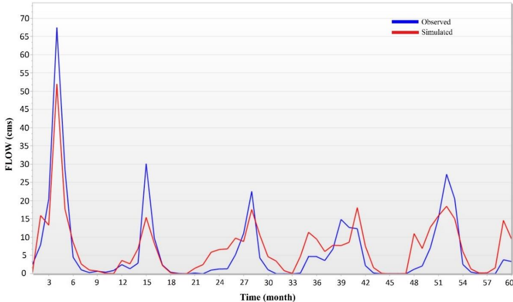
شکل ۶- نمودار داده‌های شبیه‌سازی شده و مشاهداتی رواناب ماهانه در سال‌های ۲۰۰۷ تا ۲۰۱۱ (مرحله واسنجی مدل) Fig. 6 Diagram of simulated data and monthly runoff observations for 2007-2011 (model calibration step)
