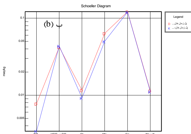
شکل ۷- تفاوت مقادیر یون‌ها (الف) در ایستگاه اسکندری و (ب) ر ایستگاه پل زمان‌خان Fig. 7 Changes in ions at a) Eskandari and b) Pol-e-Zaman Khan stations
