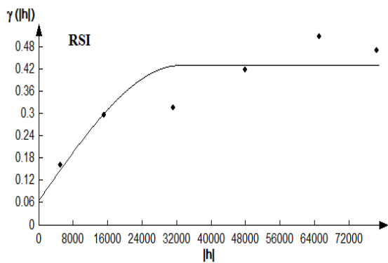
شکل ۲- واریوگرام‌های تجربی و مدل نظری برازش داده شده به شاخص‌های کیفی آب زیرزمینی دشت مرودشت
