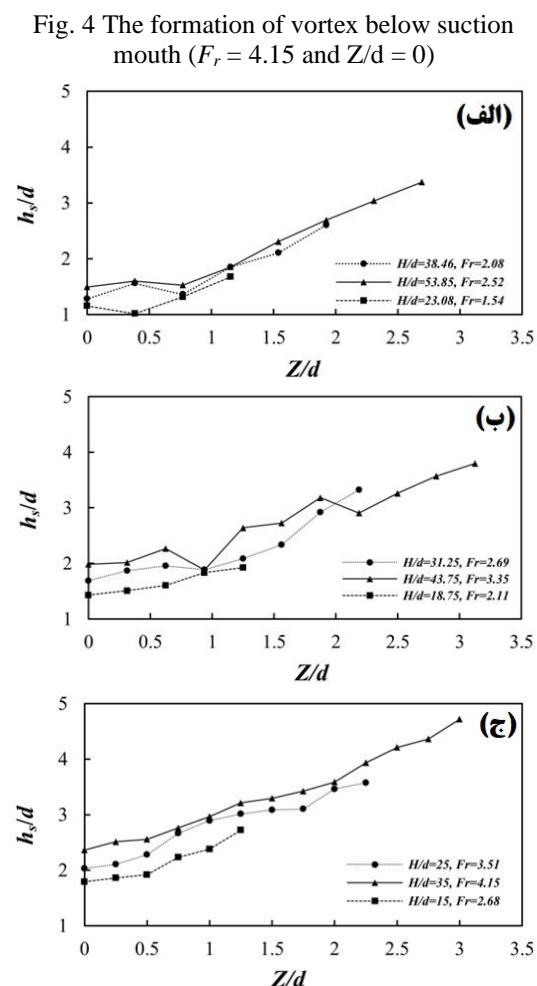
شکل ۵- حداکثر عمق حفره آبشستگی مشاهده‌شده در سیفون لایروبی در (الف) d = 13 ، (ب) d = 16 ، و (ج) d = 20 mm Fig. 5 The observed results for the maximum scour depth of the hydro-suction system at a) d = 13 , b) d = 16 , and c) d = 20 mm
